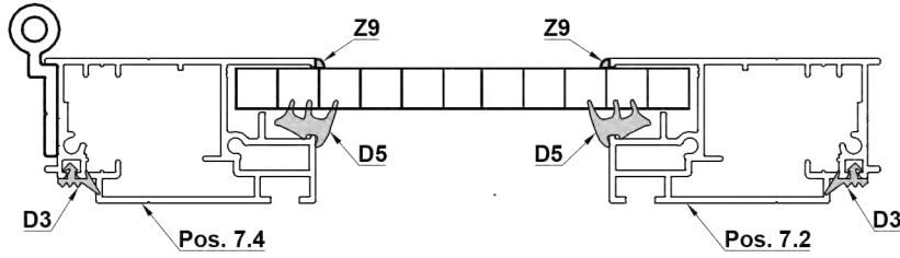
Detail A-A
